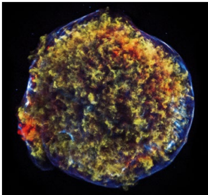
Fig.3. Image composite en rayons X du reste de la supernova de Tycho observée par le satellite Chandra. Les couleurs représentent différentes bandes d'énergie. En rouge (0,95-1,26 keV), l'émission est dominée par les raies d'émission du fer ; en vert (1,63-2,26 keV) par celles du silicium et en bleu par le continu à haute énergie (4,1-6,1 keV). La taille apparente du reste est de 8 minutes d'arc. Crédit : NASA/CXC/SAO.
