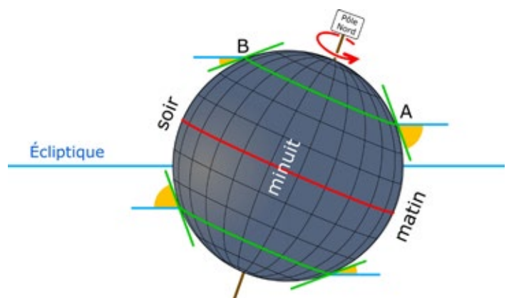
Fig.4. La Terre à l'équinoxe de septembre. Le Soleil est situé derrière la Terre. On a représenté quatre horizons en vert aux latitudes 45^\circ N et 45^\circ S, aux levers et couchers du Soleil.
