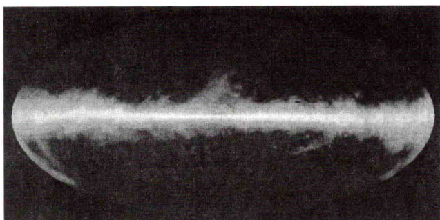
fig. 1 : vue du ciel à la longueur d'onde de 21 cm
