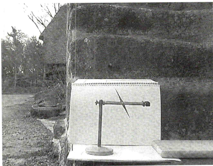
Photo n° 6 : inclinaison magnétique à Bubry (Bretagne)
