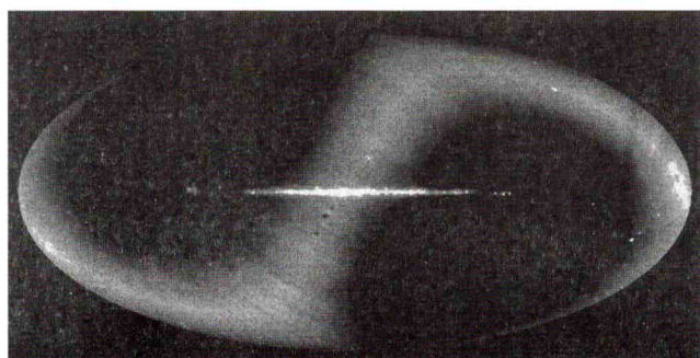
fig. 5 : l'écliptique trahi par les poussières qu'il contient
