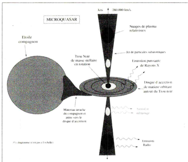
fig. 3 : vue schématique du microquasar GRS1915+105
