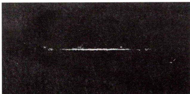
fig. 2 : vue du ciel à la longueur d'onde du CO
