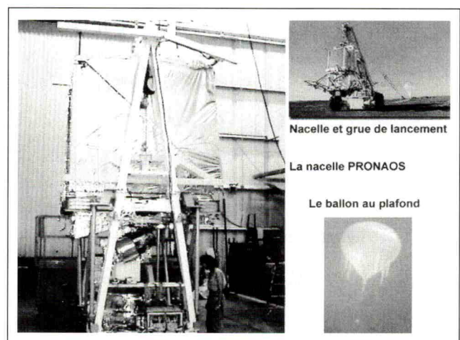
fig. 4 : l'expérience PRONAOS (à gauche), prête à décoller à Fort Sumner, Nouveau-Mexique et prise en photo au plafond.
