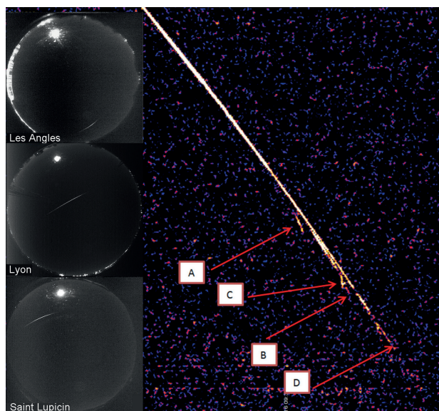
Fig.5. Détection du bolide du 22 juin 2016.
