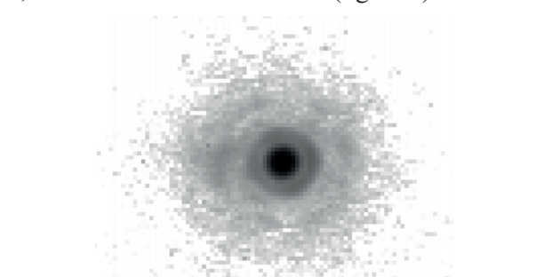
Fig.3. Image d'une étoile dans le proche infrarouge, fournie par un des télescopes auxiliaires du VLT (AT) et corrigée par l'optique adaptative MACAO de celui-ci. Le rapport de Strehl vaut ici S = 0,62 . Outre l'image centrale, on distingue le premier et le second anneau de la figure de diffraction (figure d'Airy) (Document N. Hubin, ESO).
