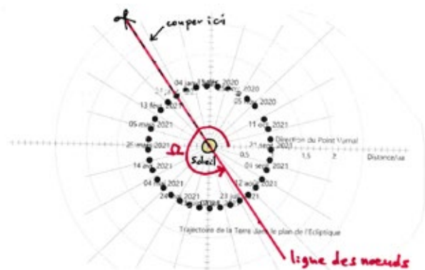
Fig. 9b. Orbite de la Terre.
