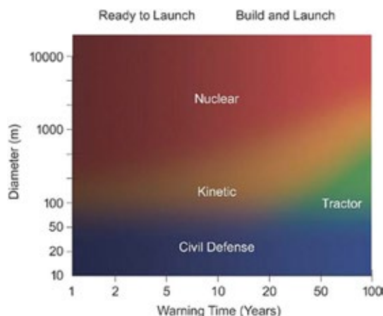
Fig.5. Comparaison entre quatre types de techniques de défense planétaire en fonction du diamètre de l'astéroïde et du temps restant pour réagir (crédit Tim Warchocki).
