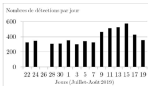
Fig.9. Nombre de météores détectés journalièrement durant les Perséides avec cette instrumentation. Le nombre de météores augmente lors du pic d'activité (11-15 août) à environ 30 détectés par heure.
