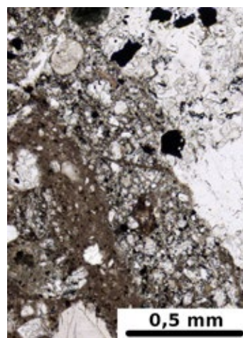
Fig.5. Échantillon Apollo 14267. Photographie de l'échantillon et photographie d'une lame mince de l'échantillon. Cette roche est une brèche d'impact. On observe les clastes à l'échelle macroscopique, mais aussi microscopique (source : NASA).
