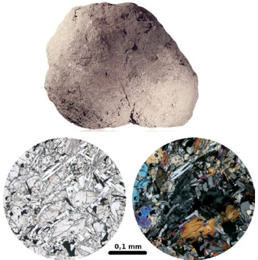
Fig.7. Photographies macroscopique et microscopique de l'échantillon Apollo 12002. Ce basalte est composé de clinopyroxènes, olivine et plagioclase. (source NASA).
