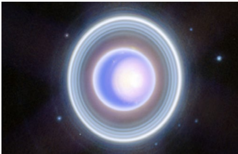
Fig.4. Image réalisée par l'instrument NIRCам du télescope James Webb où l'on voit le pôle Nord de la planète, les groupes d'anneaux principaux \epsilon , \delta\gamma\eta , \beta\alpha , 456 et \zeta (de l'extérieur vers l'intérieur). On distingue d'autres anneaux extérieurs ainsi que 9 des 27 lunes connues d'Uranus.
