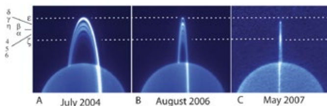
Fig.3. Images des anneaux d'Uranus prises par le télescope Keck II en 2004 et 2006 avant le passage de la Terre et du Soleil dans le plan des anneaux (deux images de gauche) et le 28 mai 2007, au moment où la Terre est du côté non éclairé des anneaux (à droite). Les pointillés indiquent la position des anneaux \epsilon (ligne supérieure) et \zeta (ligne inférieure), les autres anneaux étant indiqués. Imke de Pater (UC Berkeley), Heidi B. Hammel (SSI, Boulder) et l'Observatoire W. M. Keck.
