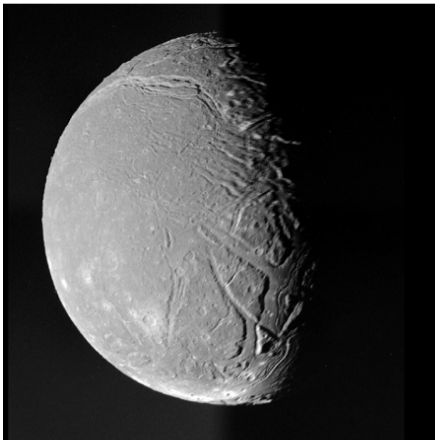
Fig.5. Mosaïque des quatre images à haute résolution faite du satellite Ariel par Voyager 2 le 24 janvier 1986. La résolution est de 2,4 km, le diamètre du satellite est d'environ 1 200 km. Les failles visibles auraient été produites par l'étirement de la croûte sous les effets de marée.
