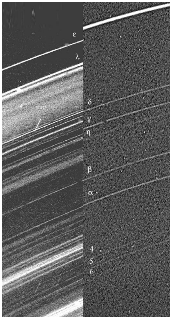
Fig.2. Image composite des principaux anneaux d'Uranus en lumière diffusée vers « l'avant » (à gauche) et en rétrodiffusion (à droite). L'image de gauche est la seule image des anneaux d'Uranus prise avec un angle de phase élevé par Voyager 2. Ces images montrent que les anneaux principaux denses sont entrelacés avec un réseau de structures de poussière. L'origine de cette structuration est inconnue. Crédit photo : NASA/JPL.
