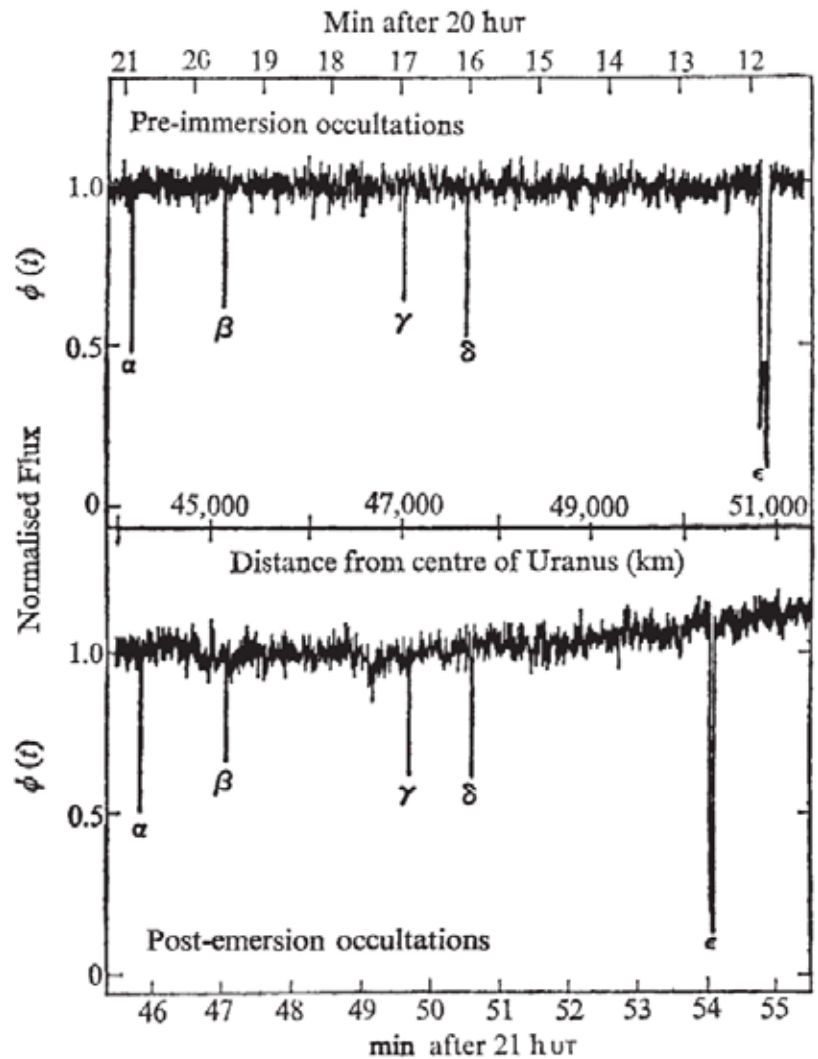
Fig.1. Luminosité de l'étoile observée à partir de l'observatoire aéroporté Kuiper en 1977 alors qu'Uranus s'approchait d'elle, montrant des baisses brutales lorsque cinq des anneaux étroits d'Uranus ont balayé l'étoile telle que vue de l'observatoire. Adapté d'Elliott et al. (1977).
